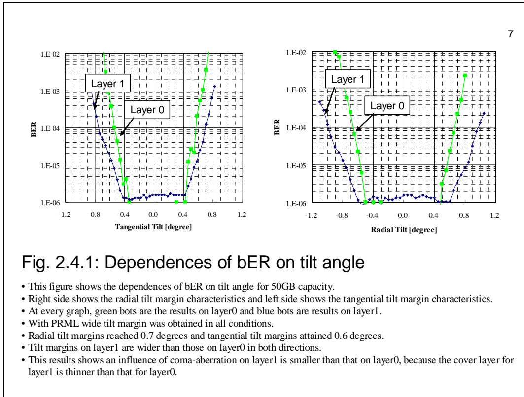
Fig. 2.4.1 Tilt margins
