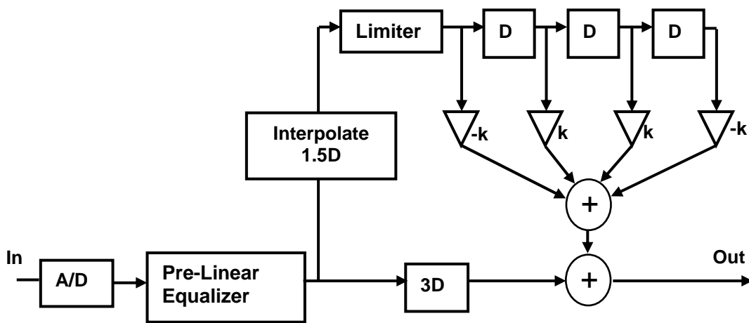
Fig. 2.5.2 Configuration of the Limit-EQ
